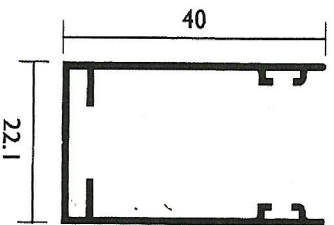
DETAIL ZIJDELEIDER / DETAIL COULISSES LATÉRALES
